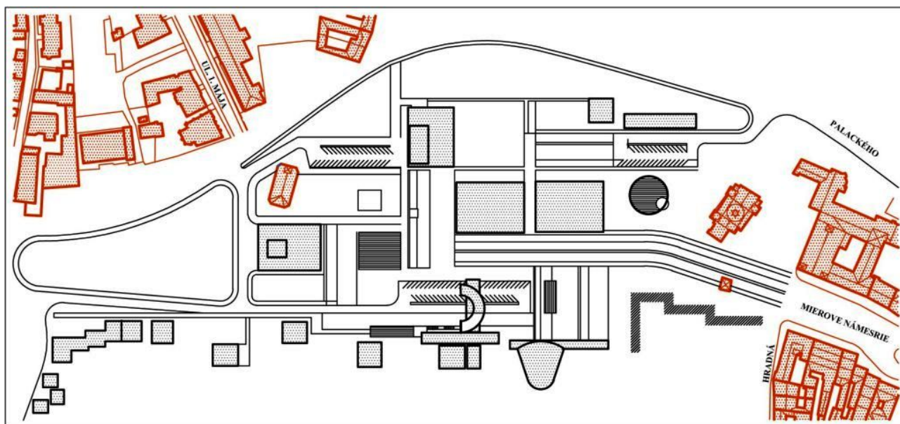
URBANISTICKÁ ŠTÚDIA – TRENČÍN PREDMOSTIE. Ing.arch. Blicha, konzultant Krajíček, 1966
